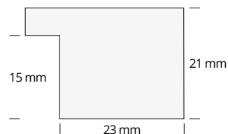
Sezione cornice dimensioni reali Frame section real sizes
